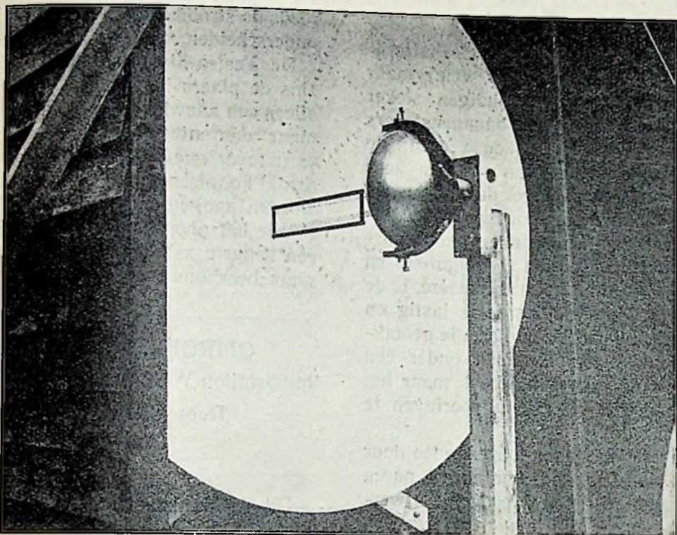
Fig. 6. De ontvanger: het verste verticale been van het rechthoekige raampje is de ontvangdipool.
