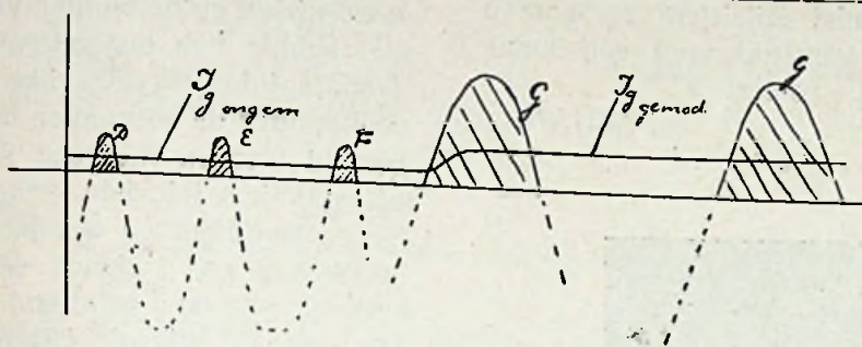
Fig. 2. Het verloop van den roosterstroom in ongemoduleerden en in gemoduleerden toestand, afgeleid uit fig. 1.
