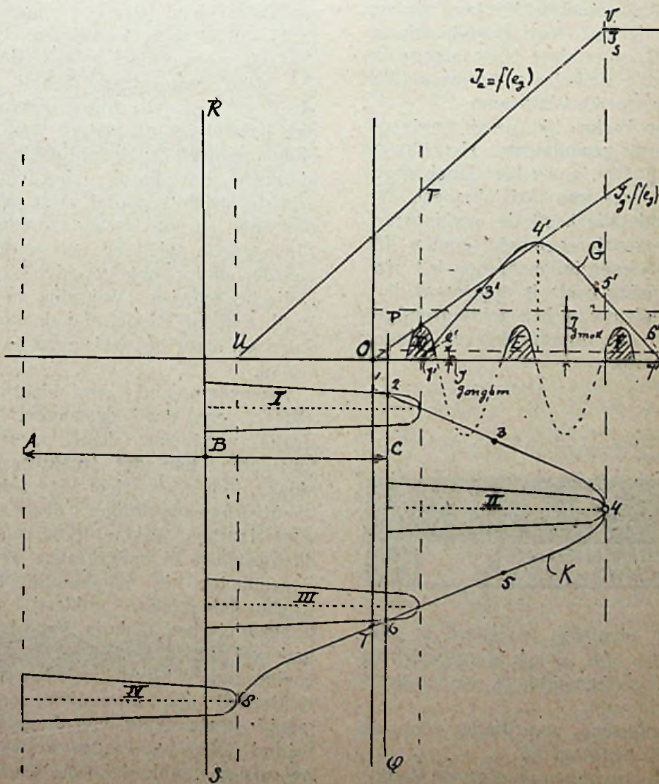
Fig. 1. Het verloop van de rooster spanningen en stroomen in de zendlamp.
