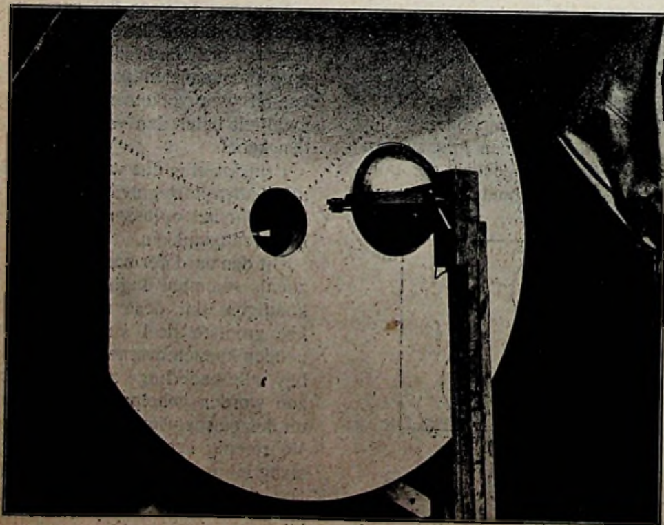
Fig. 5: De zender; het dipoolantennetje is juist even zichtbaar aan den houder, links van den kleinen, halve-bolvormigen spiegel.
